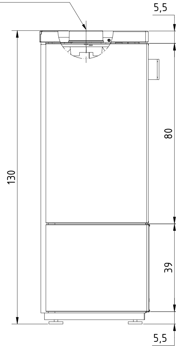
Rauchrohranschluss Ø15 Seite
